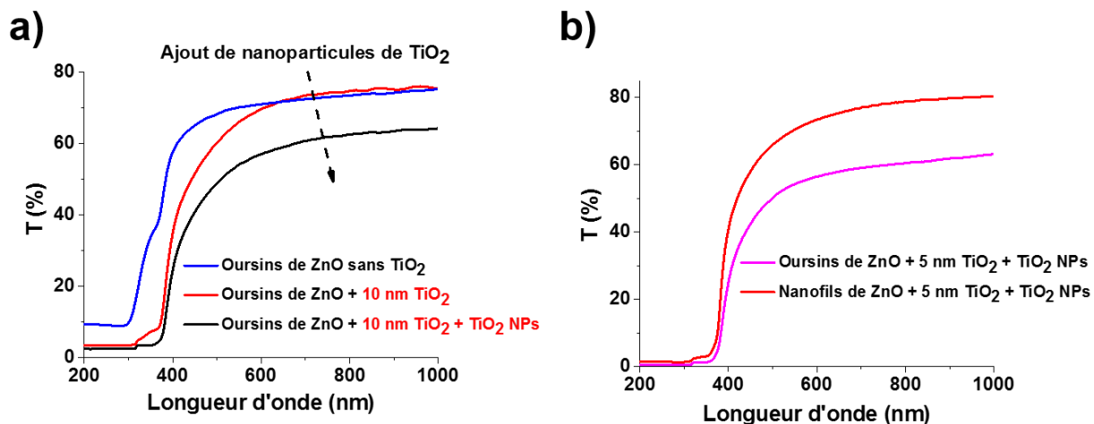
Figure III.14: Spectres de transmittance (a) des oursins de ZnO et de la structure cœur / coquille formée de l'ensemble ZnO oursins / \text{TiO}_2 10 nm couche et ZnO oursins / \text{TiO}_2 10 nm couche / \text{TiO}_2 NPs et (b) comparaison de la transmittance de lumière dans les nanofils et oursins de nanofils de ZnO avant illumination.
