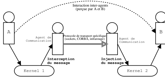
Figure 4. Agents de communication distribuée
