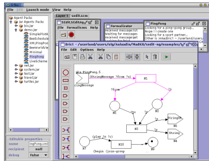
Figure 6. SEDIT, développé comme un SMA et décrivant le comportement d'un agent
