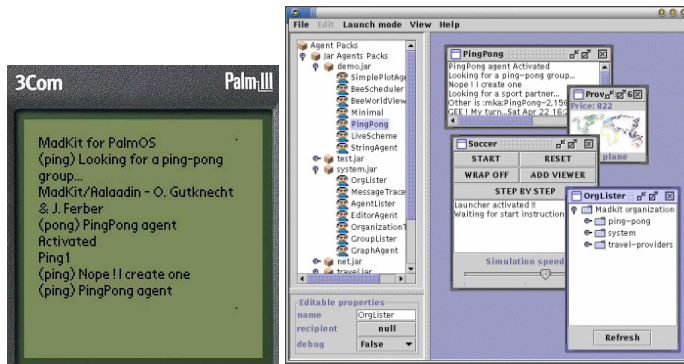
Figure 5. Des applications MADKIT dans les hôtes Palm et G-Box
