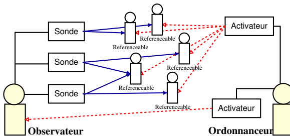
Figure 3. Fonctionnement des agents synchrones
