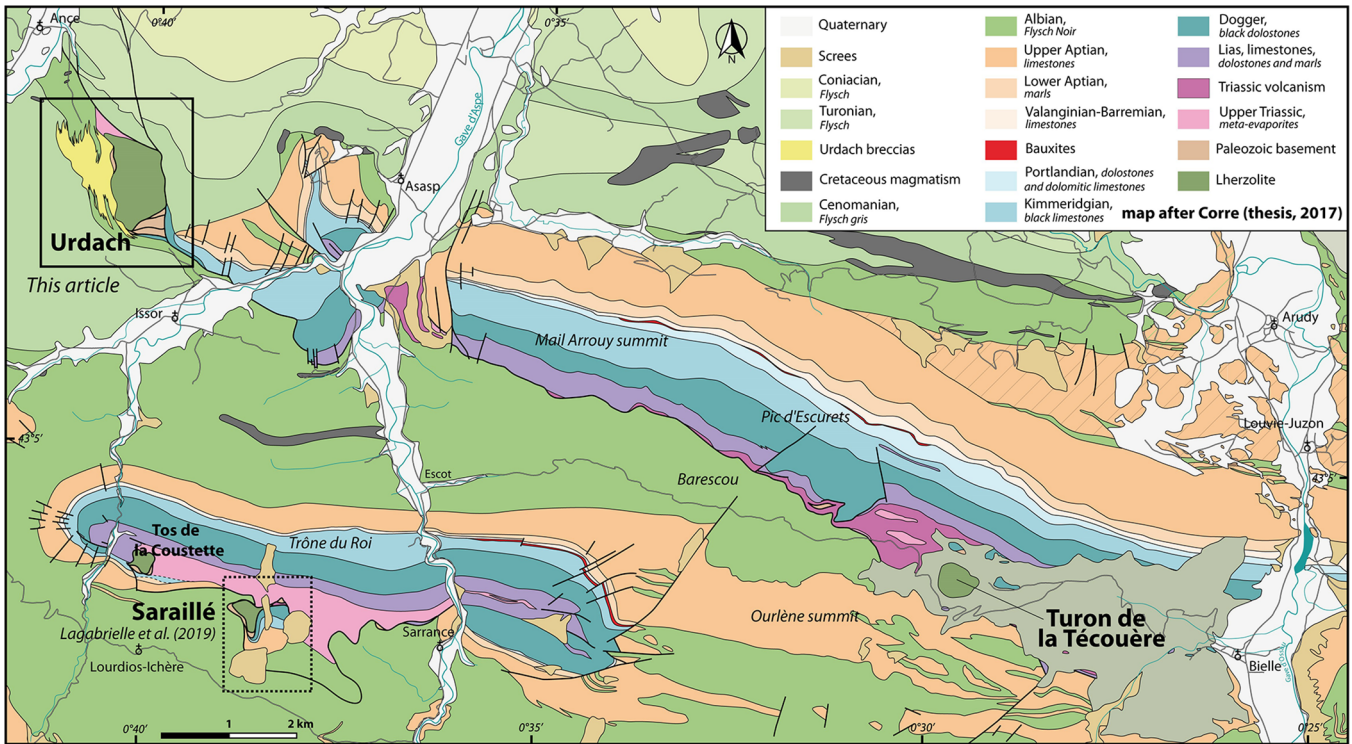
Fig. 2. Geological map of the “Chainons Béarnais” (Corre, 2017) and location of the Sarailié and Urdach lherzolite bodies. Fig. 2. Carte géologique des « Chainons Béarnais » (Corre, 2017) et situation des massifs du Sarailié et d’Urdach.
