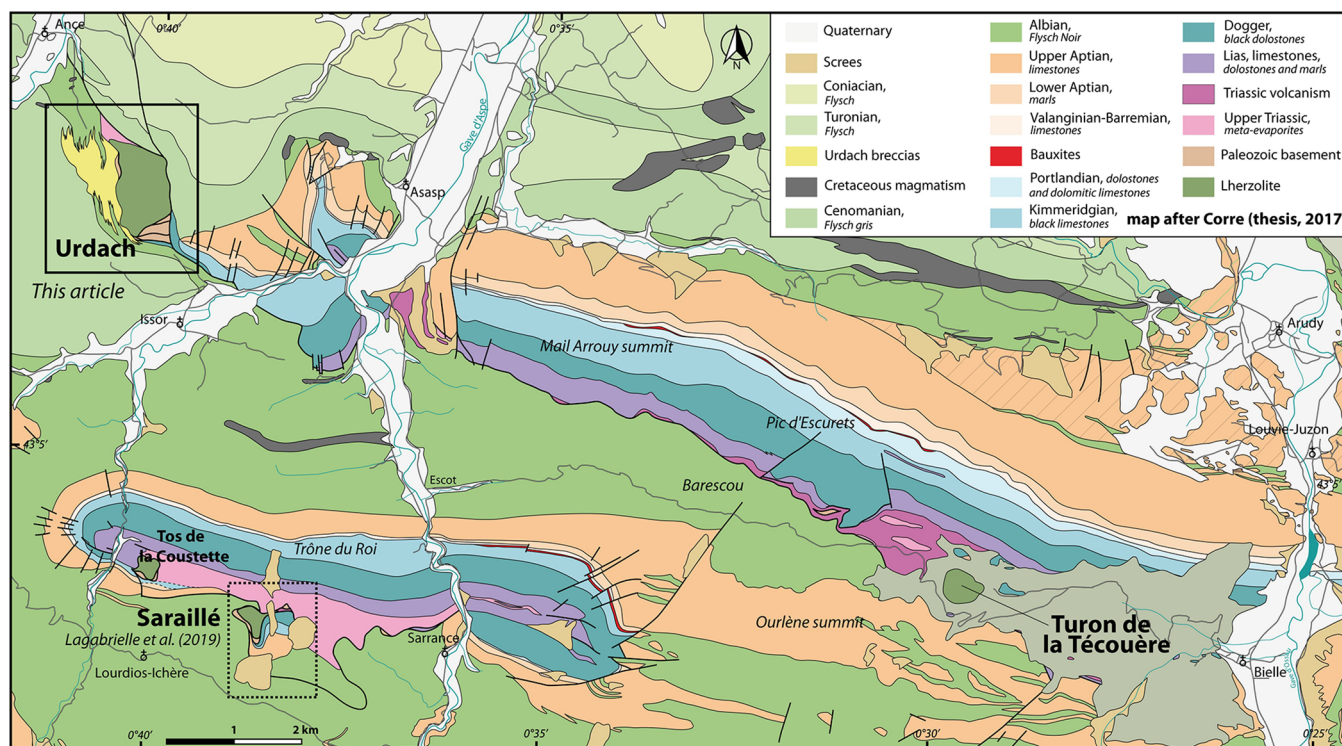
Fig. 2. Geological map of the “Chainons Béarnais” (Corre, 2017) and location of the Saraillé and Urdach lherzolite bodies. Fig. 2. Carte géologique des « Chainons Béarnais » (Corre, 2017) et situation des massifs du Saraillé et d’Urdach.
