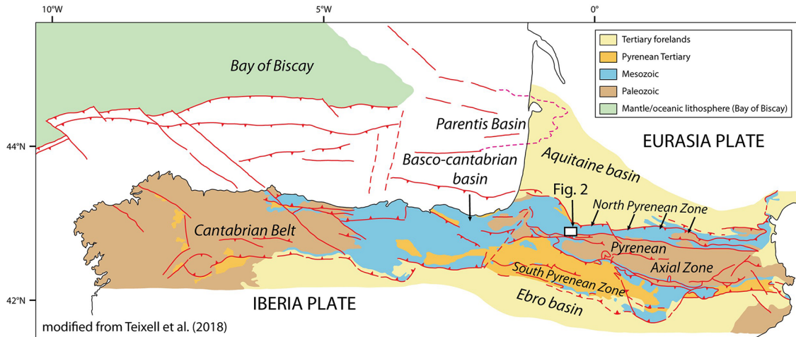
Fig. 1. Simplified structural map of the Pyrenean-Cantabrian belt and location of the study area (modified after Teixell et al. , 2018 ). Fig. 1. Carte simplifiée de la chaîne Pyrénéo-cantabrique et localisation de la zone étudiée (modifiée d'après Teixell et al. , 2018 ).
